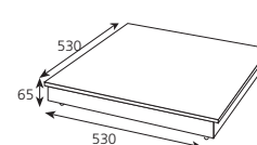
PC-5050-E Modelo encastrable con mando remoto incluido
