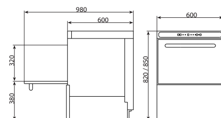
Dimensiones de los modelos AF-540, AF-540-B, AF-720 y AF-720-B
