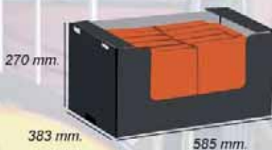
cajas expositoras de cuarto de palet europeo
