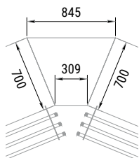
MUEBLE ANGULAR CERRADO 45° SELF INFANTIL
