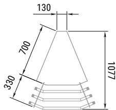
MUEBLE ANGULAR ABIERTO 45° SELF INFANTIL
