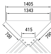
MUEBLE ANGULAR CERRADO 90° SELF INFANTIL
